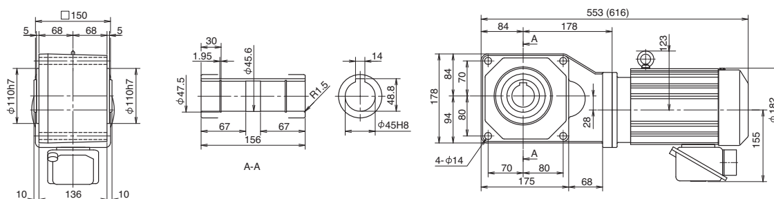
Fig. 5 RNYM3-1520-5~30 (RNYM3-1520-B-5~30) Mass 34kg (Mass 39kg)
