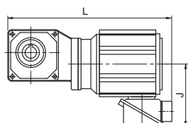
Fig. 1 0.1kW Without brake
