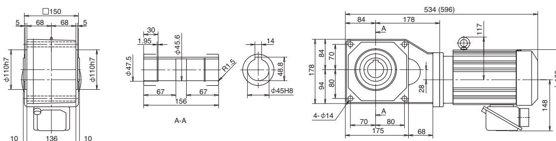
Fig. 6 RNYM2-1520-5~10 (RNYM2-1520-B-5~10) Mass 31kg (Mass 35kg)
