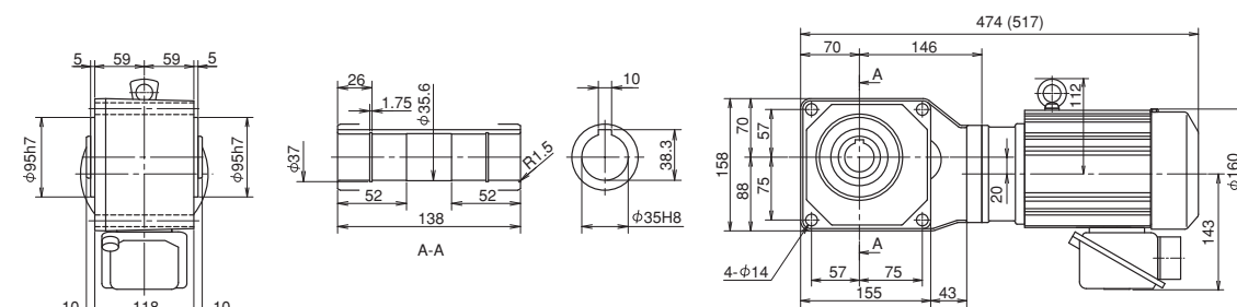
Fig. 5 RNYM08-1420-40-60 (RNYM08-1420-B-40-60) Mass 17kg (Mass 19kg)
