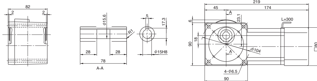
Fig. 2 RNYM004-17-CC-150~240 Mass 4.1kg
