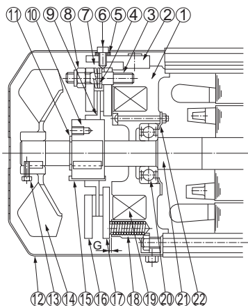
Fig. 25 FB-10B, 15B (7.5~11kW×4 poles)
