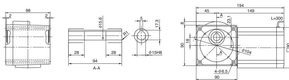
Fig. 2 RNYM004-17-CC-150~240 Mass 4.1kg
