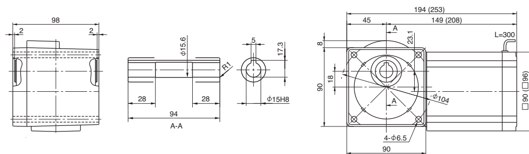
Fig. 2 RNYM004-17-150~240 (RNYM004-17-B-150~240) Mass 3.7kg (Mass 4.1kg)
