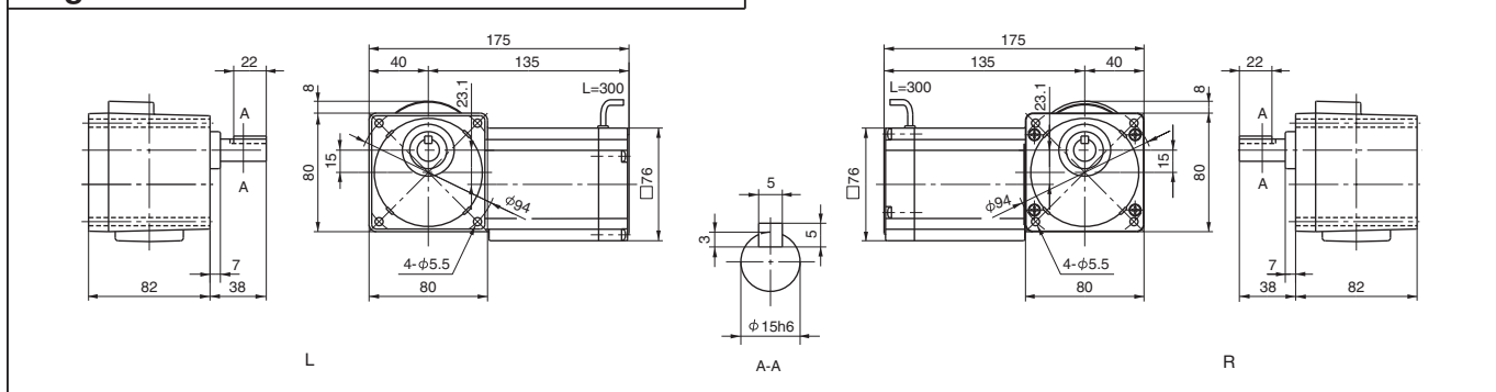
Fig. 2 RNFM0015-03 1/2-CC-120~240 Mass 2.7kg
