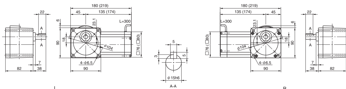
Fig. 5 RNFM006-17 L-80~240 Mass 4.0kg (RNFM006-17 R-B-80~240) (Mass 4.4kg)
