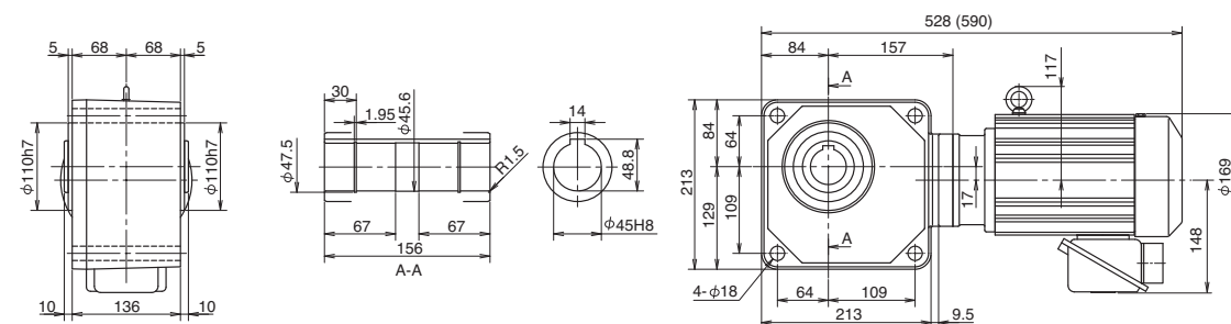
Fig. 4 RNYM2-1531-40-80 (RNYM2-1531-B-40-80)
