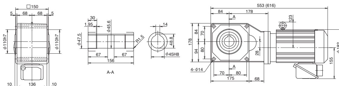
Fig. 6 RNYM3-1521-5~25 (RNYM3-1521-B-5~25) Mass 34kg (Mass 39kg)
