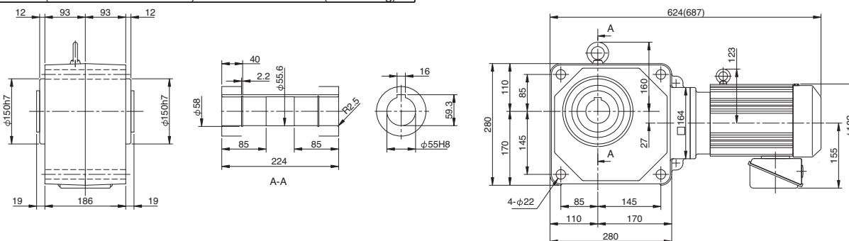
Fig. 2 RNYM3-1632-30-60 (RNYM3-1632-B-30-60) Mass 55kg (Mass 61kg)
