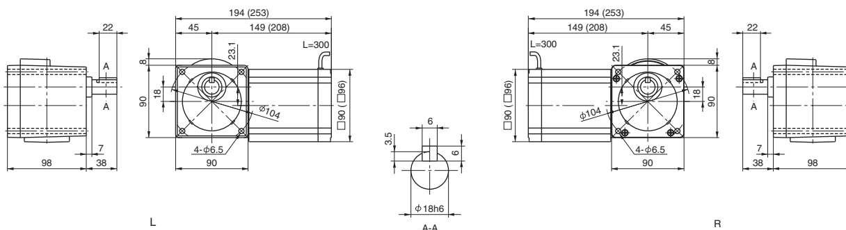
Fig. 5 RNFM006-17 L-80~240 Mass 4.0kg (RNFM006-17 R-B-80~240) (Mass 4.4kg)
