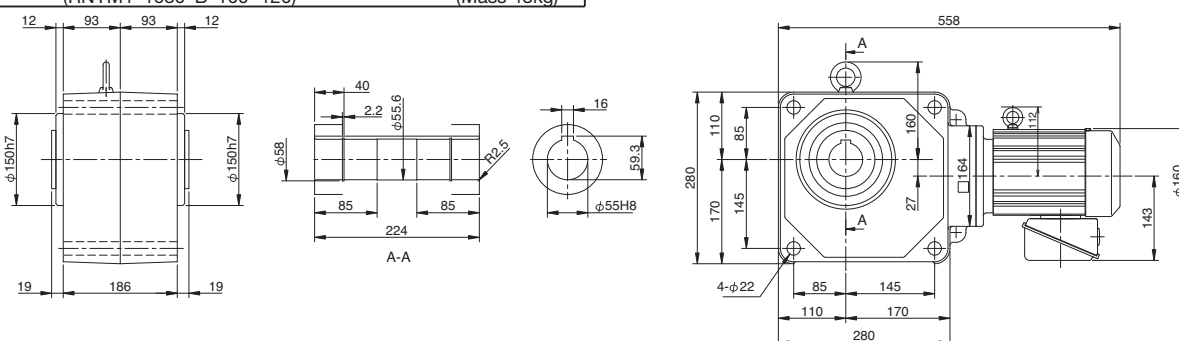
Fig. 6 RNYM1-1630-100-120 Mass 46kg (RNYM1-1630-B-100-120) (Mass 48kg)
