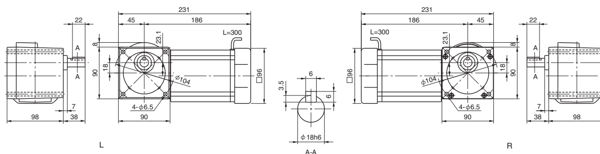
Fig. 5 RNFM006-17 \frac{1}{2} -CC-80-120 Mass 4.9kg
