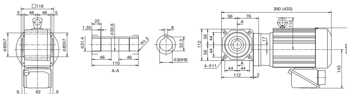
Fig. 3 RNYM08-1310-5-10 (RNYM08-1310-B-5-10) Mass 12kg (Mass 14kg)
