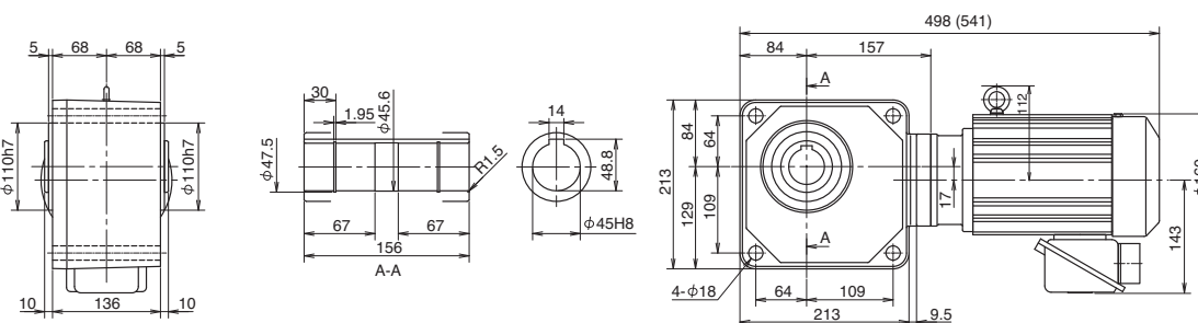
Fig. 5 RNYM1-1531-80 Mass 26kg (RNYM1-1531-B-80) (Mass 28kg)
