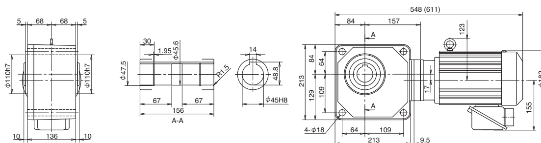
Fig. 3 RNYM3-1531-40-60 (RNYM3-1531-B-40-60) Mass 34kg (Mass 39kg)
