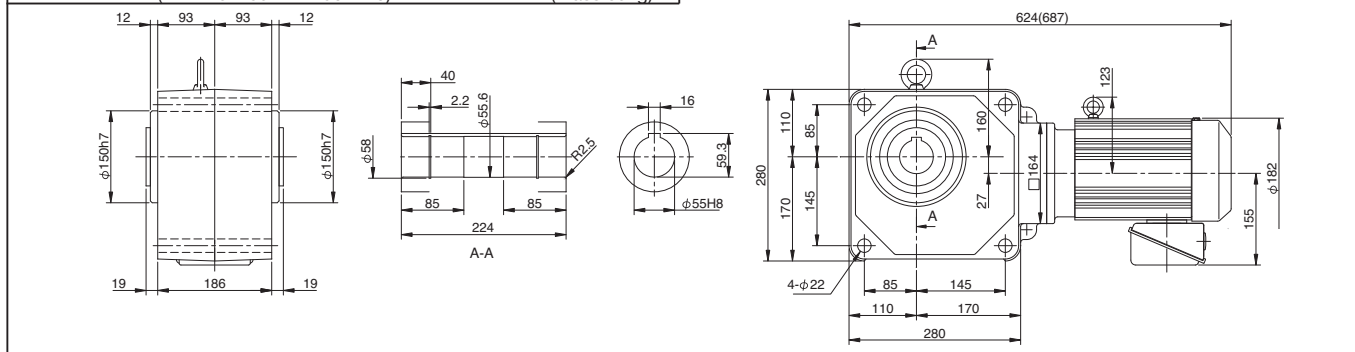
Fig. 5 RNYM3-1631-150~240 (RNYM3-1631-B-150~240) Mass 57kg (Mass 63kg)
