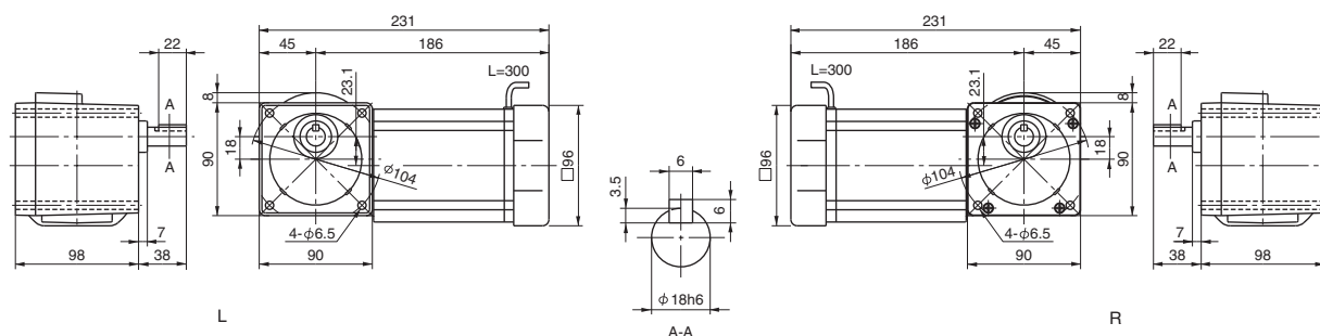
Fig. 2 RNFM009-17 \frac{1}{2} -CC-80-120 Mass 5.4kg
