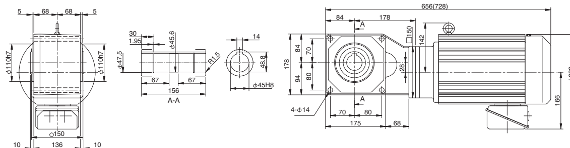
Fig. 3 RNYM5-1522-AV-5~15 (RNYM5-1522-AV-B-5~15) Mass 57kg (Mass 68kg)
