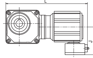
Fig. 3 0.1kW Without brake
