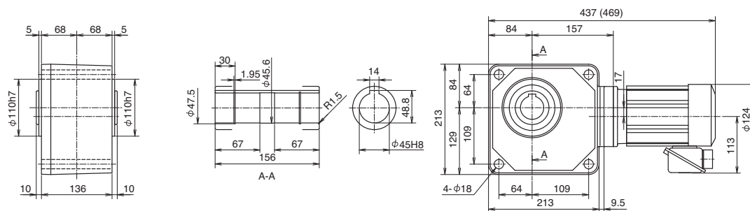
Fig. 5 RNYM05-1530-80~240 (RNYM05-1530-B-80~240) Mass 23kg (Mass 24kg)
