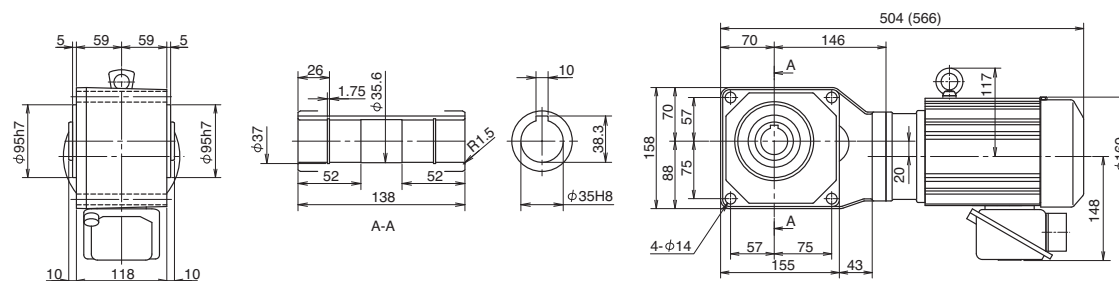
Fig. 5 RNYM1H-1420-5~30 (RNYM1H-1420-B-5~30) Mass 21kg (Mass 25kg)
