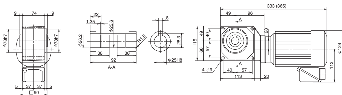
Fig. 4 RNYM01-1220-AV-40-60 (RNYM01-1220-AV-B-40-60) Mass 8.5kg (Mass 10kg)
