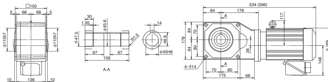
Fig. 3 RNYM2-1520-40-60 (RNYM2-1520-B-40-60)
