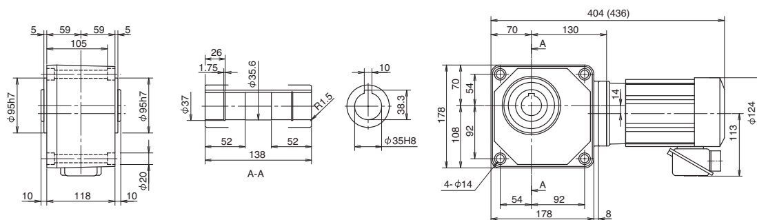
Fig. 4 RNYM05-1430-80~240 (RNYM05-1430-B-80~240) Mass 16kg (Mass 17kg)
