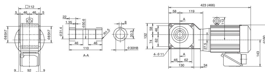
Fig. 4 RNYM08-1320-5-30 (RNYM08-1320-B-5-30) Mass 13kg (Mass 16kg)
