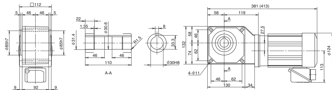
Fig. 5 RNYM03-1320-40-60 (RNYM03-1320-B-40-60) Mass 11kg (Mass 13kg)
