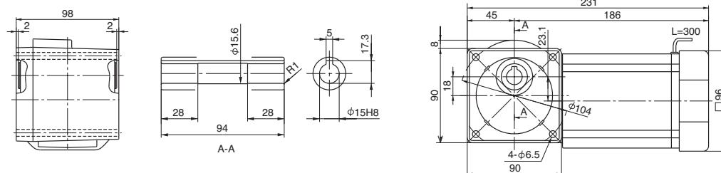
Fig. 2 RNYM009-1240-CC-300-1440 Mass 7.7kg
