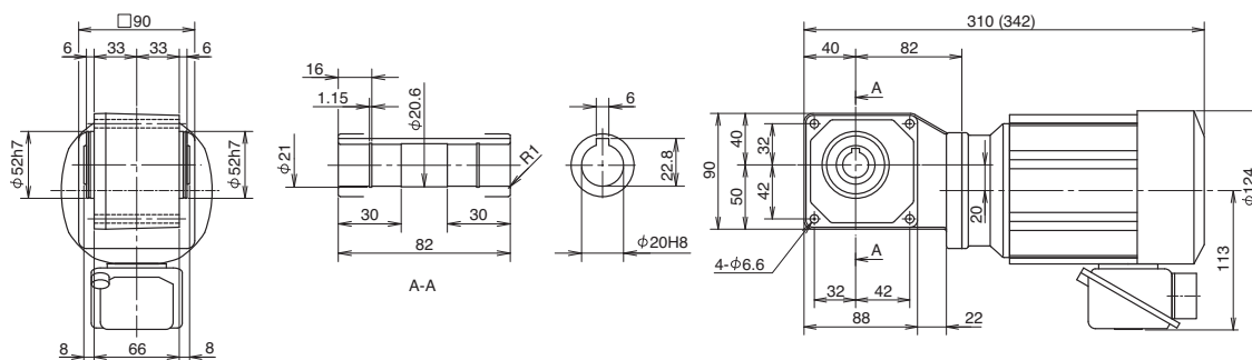
Fig. 3 RNYM01-1120-AV-5-30 (RNYM01-1120-AV-B-5-30) Mass 7.0kg (Mass 8.5kg)
