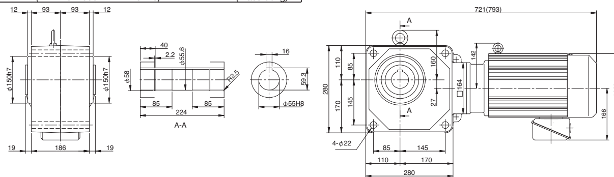
Fig. 4 RNYM5-1633-AV-20~40 (RNYM5-1633-AV-B-20~40) Mass 77kg (Mass 88kg)
