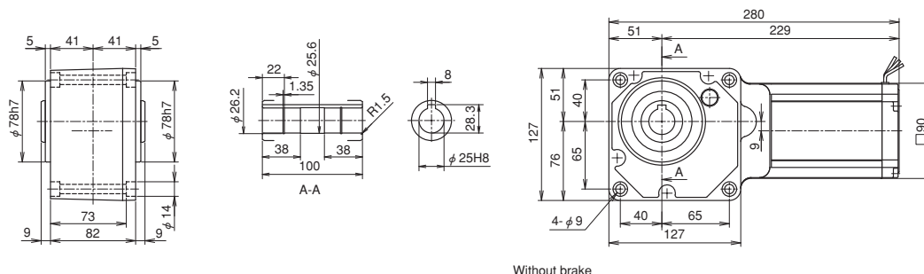
Fig. 2 RNYM009-1240-CC-300-1440 Mass 7.7kg
